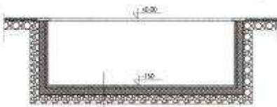
PRESJEK AA M: 1:50
